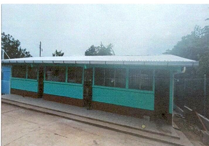
Foto 4: Mejoramiento de la cubierta metálica del Instituto (techo), con lámina troquelada No. 24 con canal para agua pluvial y bajantes fabricados en tuvos PVC.
